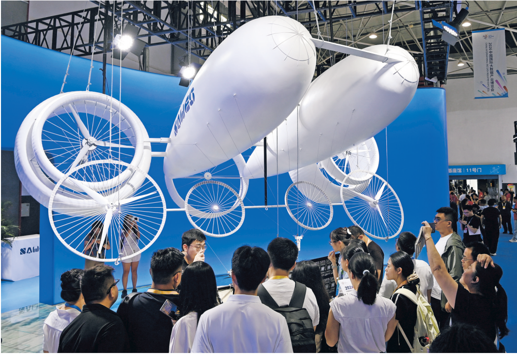
平流层浮空风力发电系统展示。
